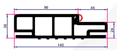
140mm KAPI KASA
