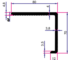
70x80 mm PERVAZ
