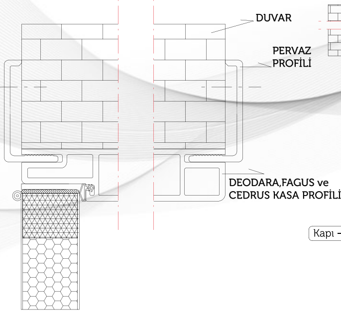
Kapı - Kasa Bağlantı Detay Üst
