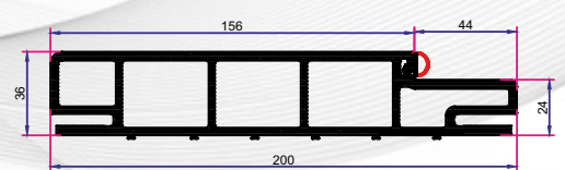
200mm KAPI KASA
