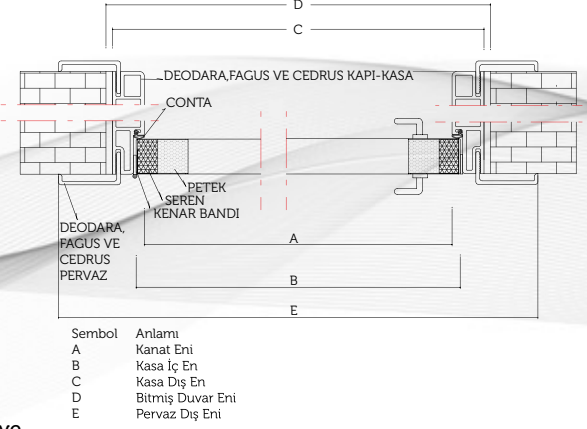
Kapı - Kasa Bağlantı Sistem Detayı
