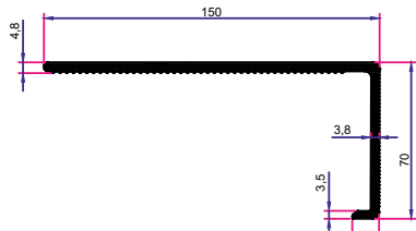
70x150 mm PERVAZ
