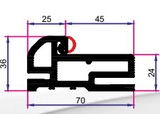
70mm KAPI KASA
